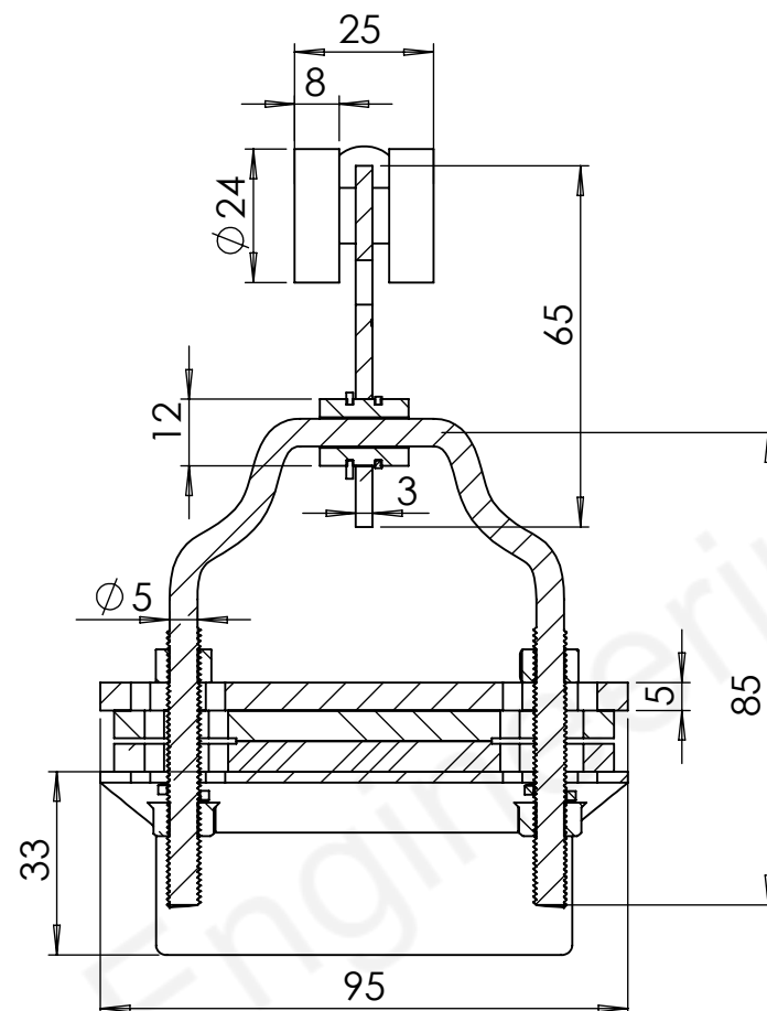
SECTION A-A SCALE 1 : 1.5
