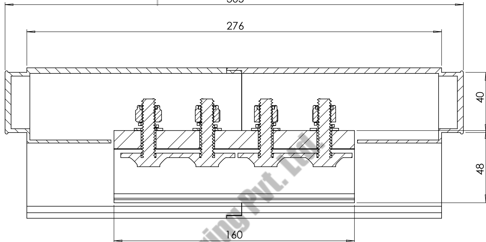
SECTION A-A SCALE 1 : 1.5
