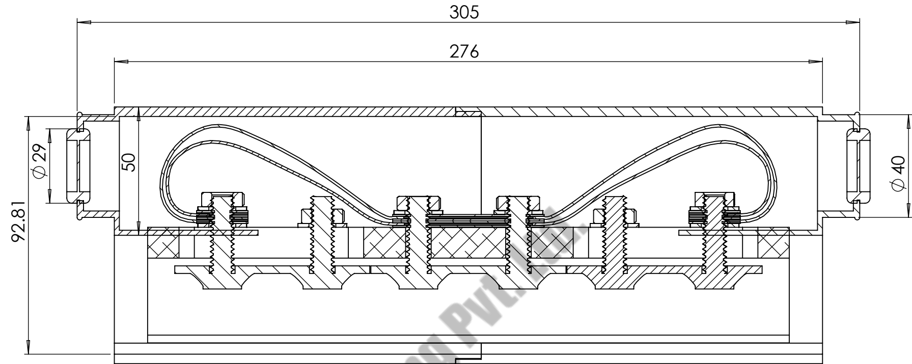
SECTION A-A SCALE 1 : 1.5
